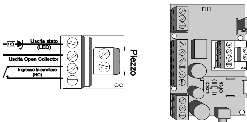
Schema 7: Collegamento scheda di espansione centrale di allarme
