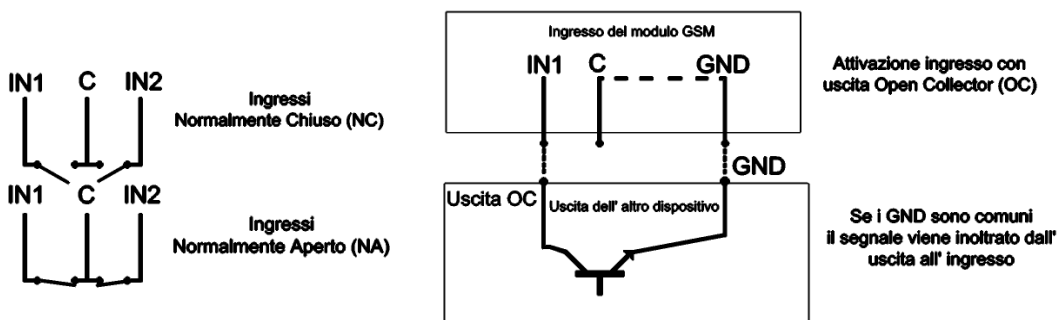
Schema 5: Collegamento Normalmente Aperto (NA) e Normalmente Chiuso (NC)
