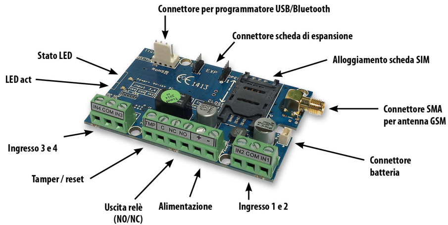
Schema 2: Struttura del dispositivo
